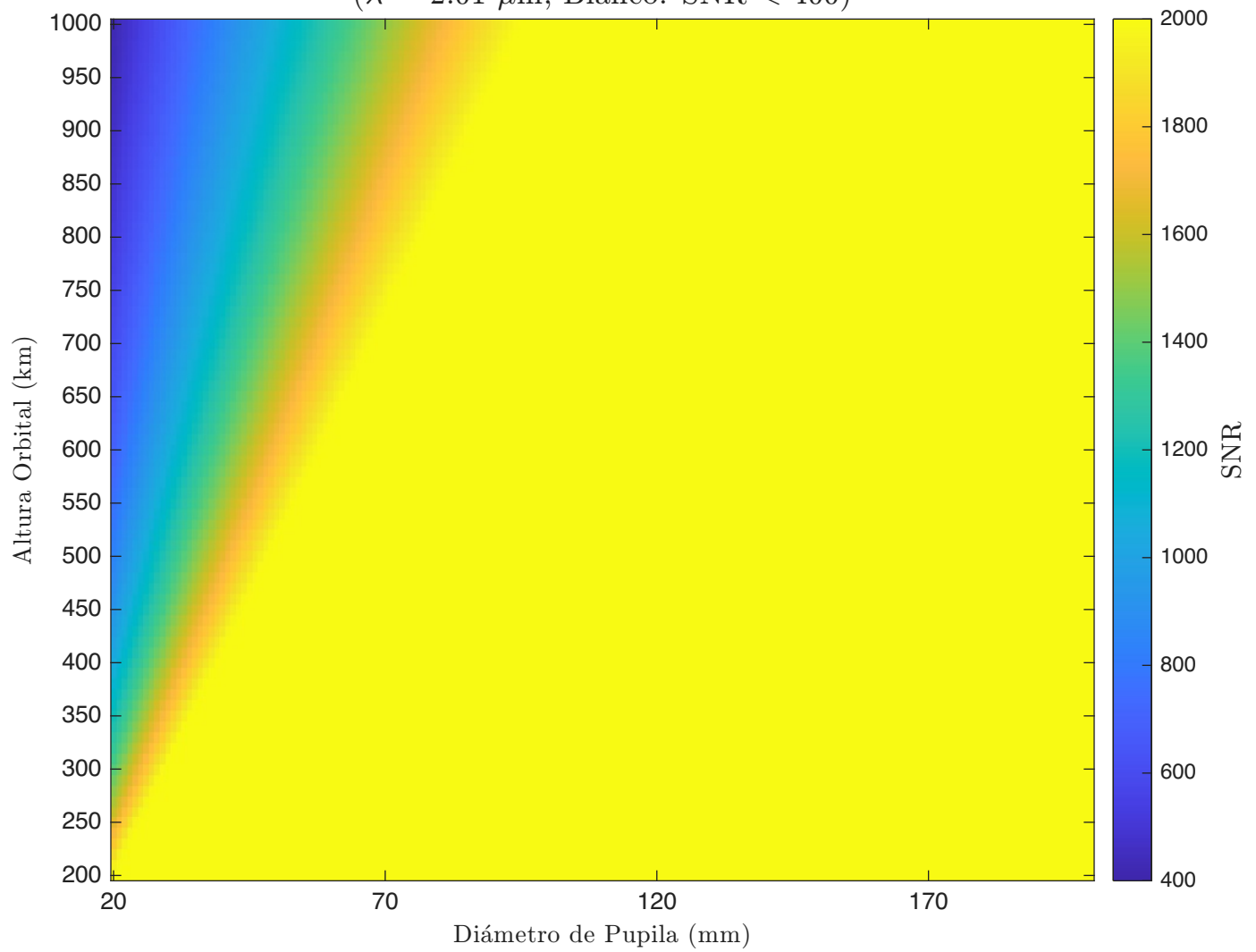
SNR - Korsch - Detector 1 ( \lambda = 2.01 \mu\text{m} , Blanco: SNR < 400)
